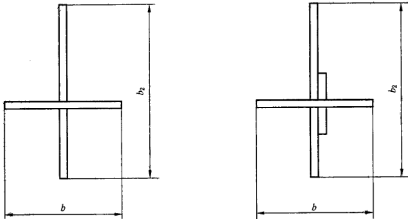
图5 测定重量偏差的典型试样
