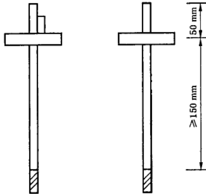
图4 抗剪试样
