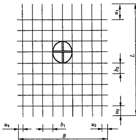
图 1 钢筋焊接网形状
